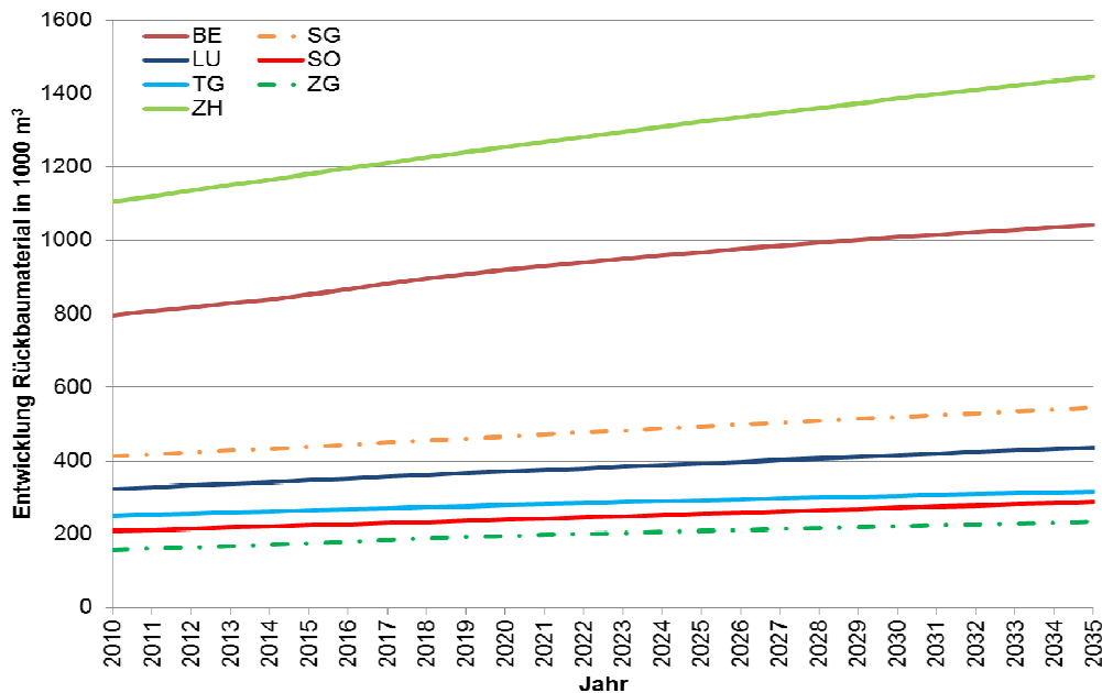
Abbildung 16: Entwicklung der neu modellierten Rückbaumaterialflüsse in den Kantonen zwischen 2010 und 2035 auf Basis der Bevölkerungsentwicklungsszenarien MITTEL des BFS. Angaben in 1000 m 3 fest.
