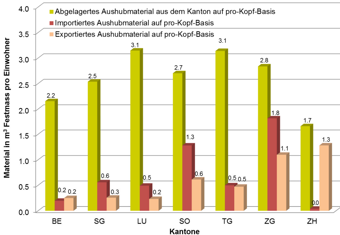
Abbildung 12: Aus den Kantonen stammende Aushubvolumina, die in den Kantonen abgelagert wurden sowie die Aushubimporte- und Exporte auf pro-Kopf-Basis für das Jahr 2013.
