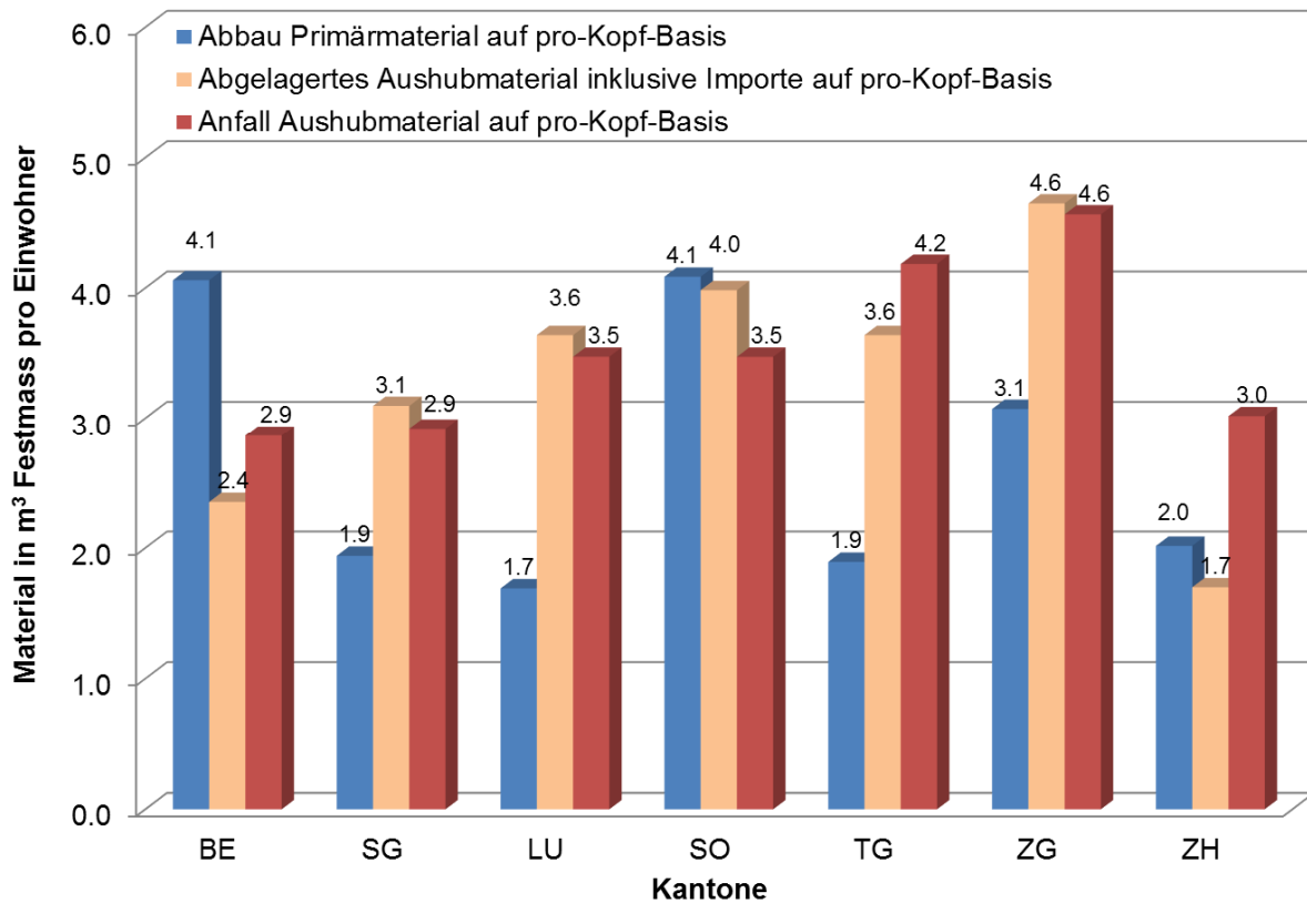
Abbildung 11: Vergleich des Primärmaterialabbaus (blaue Säulen), der Aushubablagerung inklusive Aushubimporte (hellbraun) und des Aushubanfalls (rot-braun) auf pro-Kopf-Basis für das Bezugsjahr 2013 nach Kantonen. Die Werte sind in Kubikmetern fest pro Einwohner angegeben.
