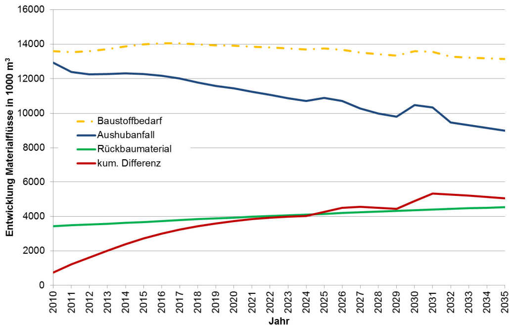
Abbildung 18: Entwicklung des Baustoffbedarfs, des Aushub- und Rückbaumaterialanfalls sowie der kumulierten Differenz zwischen Aushubablagerung und dem Primärmaterialabbau für die gesamte Region (alle sieben Kantone zusammen) zwischen 2010 und 2035. Angaben in 1000 m 3 fest.
