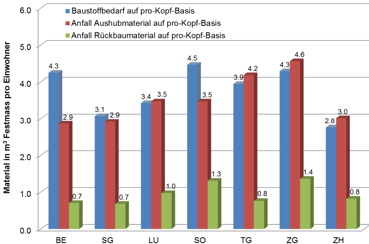
Abbildung 10: Vergleich des Baustoffbedarfs (blaue Säulen), des Aushubanfalls (braun) und des Rückbaumaterialanfalls (grün) auf pro-Kopf-Basis für das Bezugsjahr 2013 nach Kantonen. Die Werte sind in Kubikmetern fest pro Einwohner angegeben.
