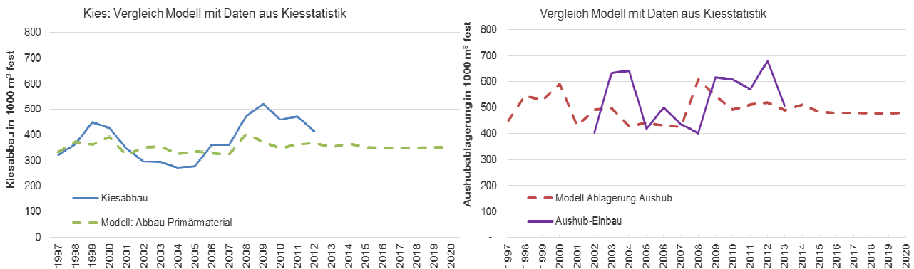
Abbildung 4: Vergleich der modellierten (gestrichelte Linien) und der tatsächlichen (ausgezogene Linien) Entwicklung des Kiesabbaus (links) und der Aushubablagerung (rechts) im Kanton Zug.
