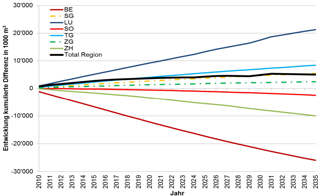
Abbildung 17: Entwicklung der kumulierten Differenz zwischen Aushubablagerung und dem Primärmaterialabbau zwischen 2010 und 2035 für das Szenario REFERENZ. Angaben in 1000 m 3 fest.
