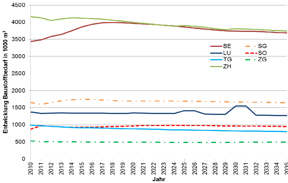
Abbildung 14: Entwicklung des neu modellierten Baustoffbedarfs in den Kantonen zwischen 2010 und 2035 auf Basis der Bevölkerungsentwicklungsszenarien MITTEL des BFS. Angaben in 1000 m 3 fest.
