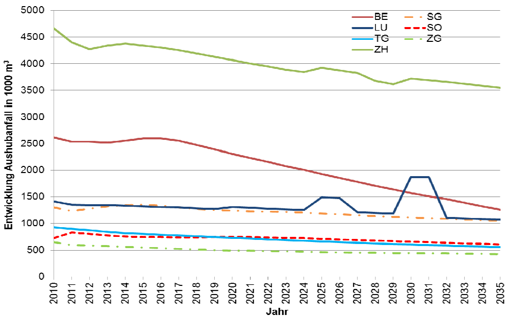
Abbildung 15: Entwicklung des neu modellierten Aushubanfalls in den Kantonen zwischen 2010 und 2035 auf Basis der Bevölkerungsentwicklungsszenarien MITTEL des BFS. Angaben in 1000 m 3 fest.
