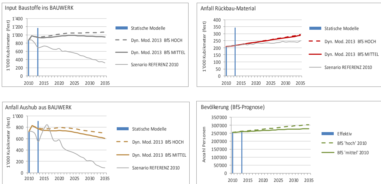
Abbildung 13: Resultate des dynamischen Modells für den Kanton Solothurn (Stand 2013, farbig) und der Vergleich mit dem Resultat REFERENZ von 2010 (grau). Die blauen Säulen zeigen die Ergebnisse der statischen Modelle 2010 und 2013. Unten rechts sind die beiden BFS-Prognosen 'mittel' und 'hoch' dargestellt.
