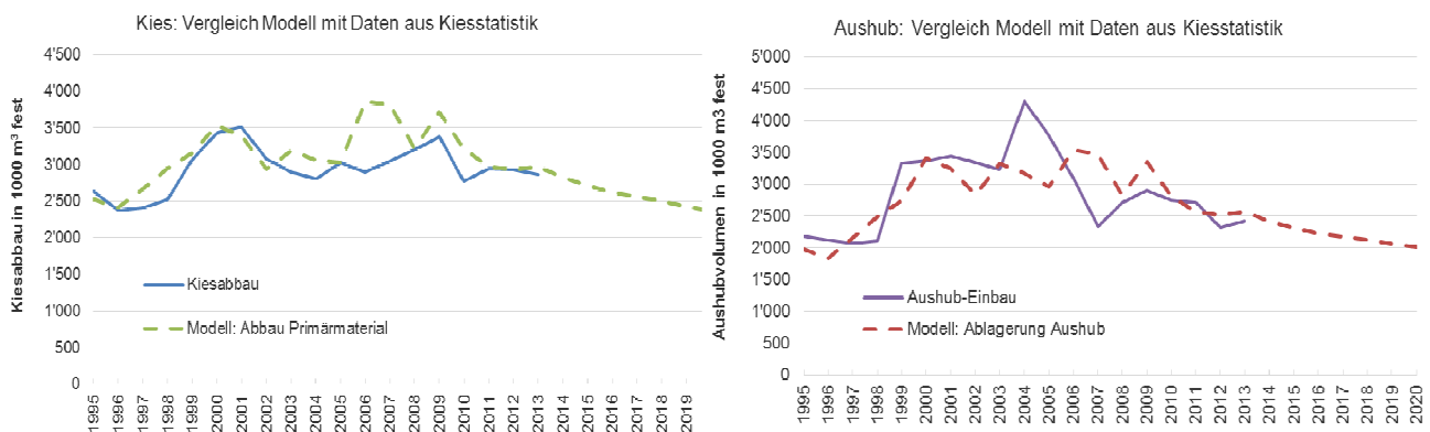
Abbildung 3: Vergleich der modellierten (gestrichelte Linien) und der tatsächlichen (ausgezogene Linien) Entwicklung des Kiesabbaus (links) und der Aushubablagerung (rechts) im Kanton Zürich.
