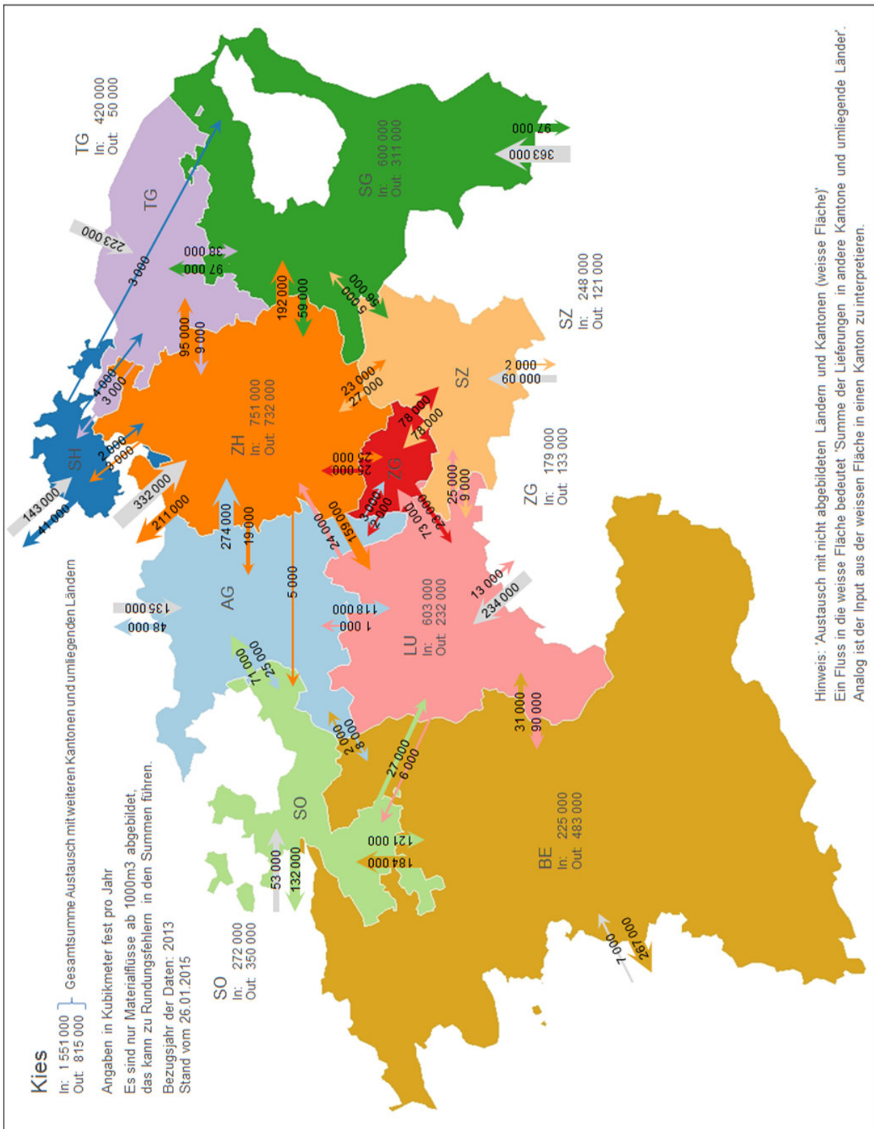
Abbildung 5: Kiesflüsse über die Kantonsgrenzen im Jahr 2013. Die Werte unterhalb den Kantonsbezeichnungen bzw. unter dem Grafiktitel «Kies» entsprechen jeweils der Summe der Importe und Exporte.
