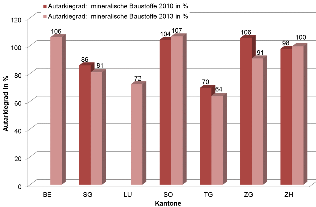
Abbildung 8: Regionale Autarkiegrade in Bezug auf die Versorgung mit mineralischen Baustoffen bzw. Kies für die Bezugsjahre 2010 und 2013. Angaben in Prozenten.
